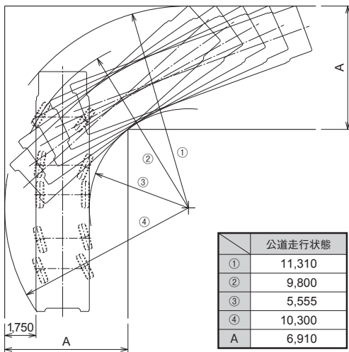
● 公道走行状態
