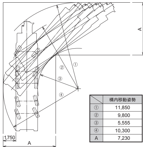
● 構内移動姿勢 (シングルトップ格納)
