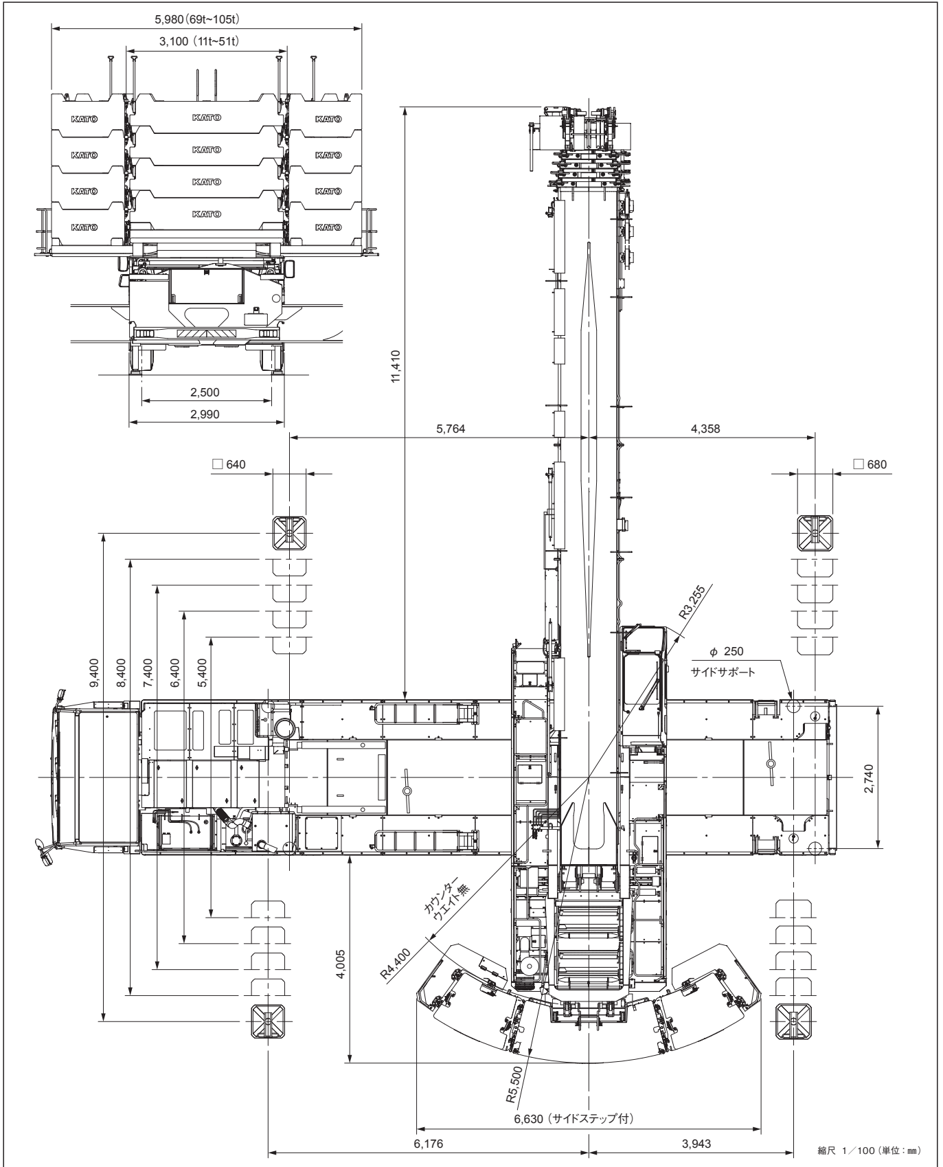
■寸法図
